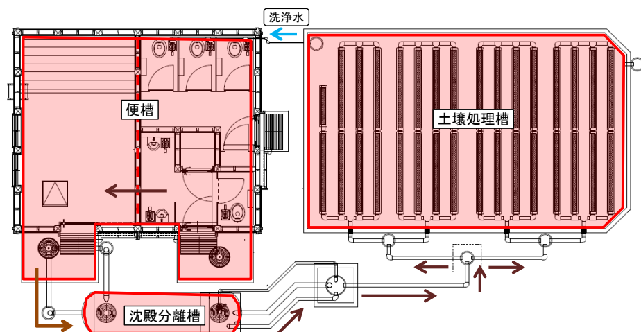
システム配置図
